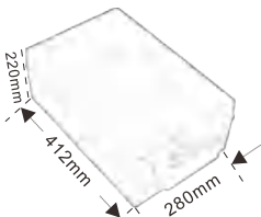
12V250AH
